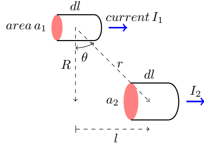
FIGURE 1. 两个水平并联导体中的两个元件 q_1, q_2 , 距离 R 分开, 角度 \theta 的角度偏移; 相应的均匀电荷密度, 电子漂移速度为 \rho_1, v_1, \rho_2, v_2 。
